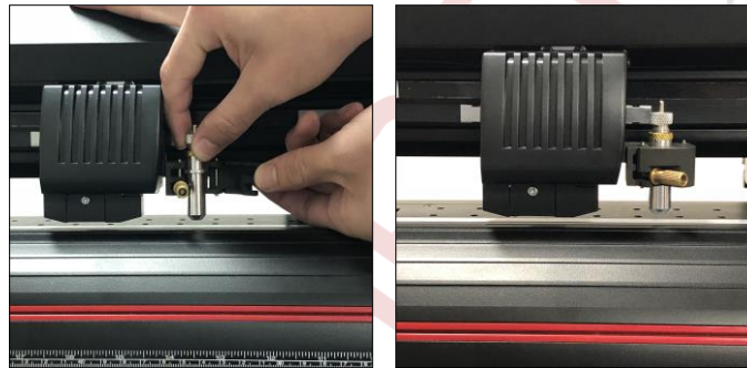
Figura 1.5 Montaje de la porta navajas en sujetador.
